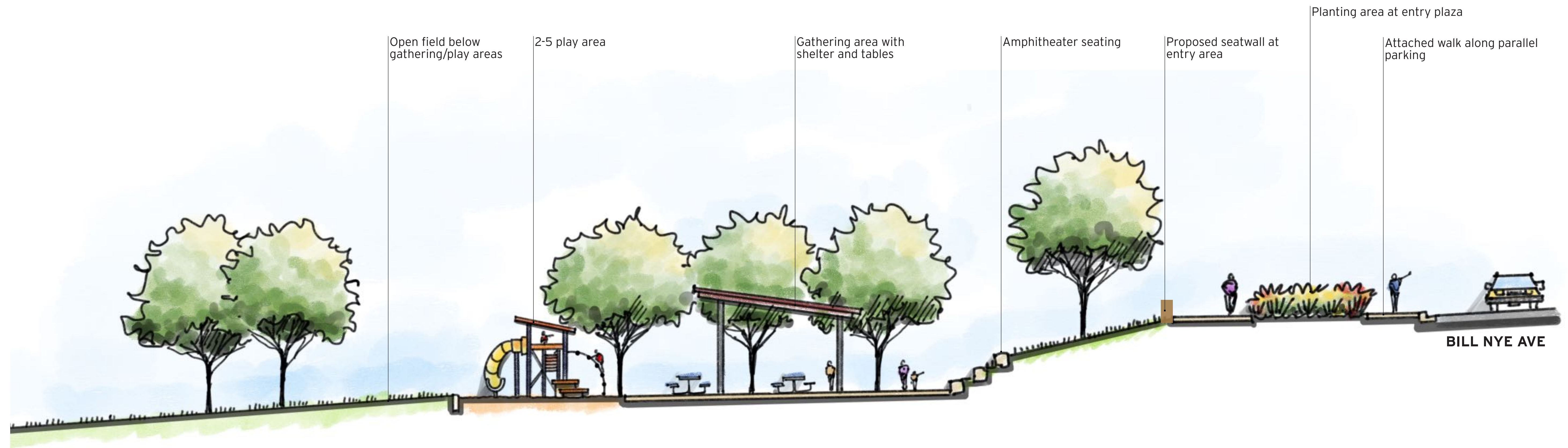
Section A-A'
